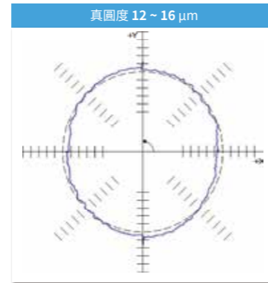
傳統滾珠螺桿機型
