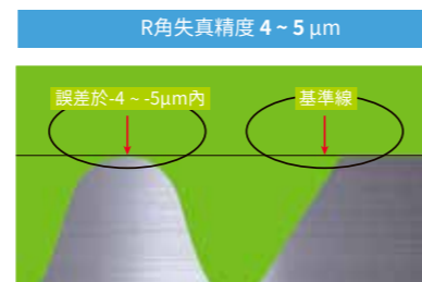
傳統滾珠螺桿機型
